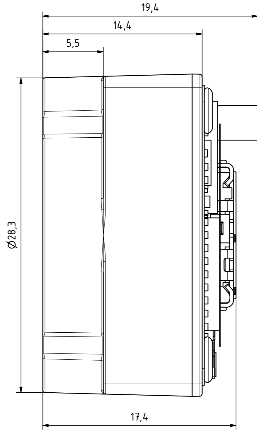
A-A ( 5 : 1 )
