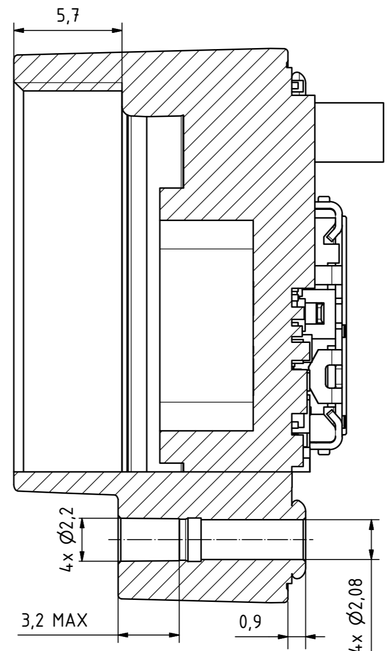
A-A ( 5 : 1 )
