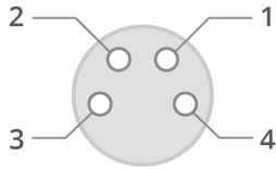
Cable side
