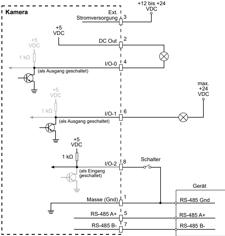
I/O-Schaltschema, Variante 1 (Eingangsschnittstelle über Schalter mit Masse (Pin 1) verbunden)
